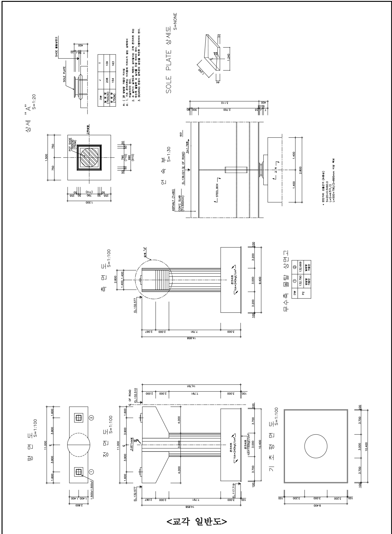
【그림 1.4.3】 홍산1교 교각 일반도
