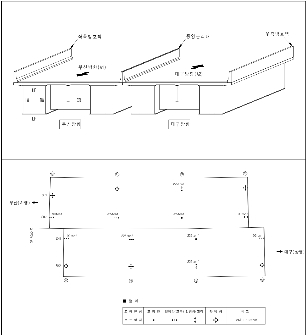
【그림 1.6.1】 교량기호의 정의
